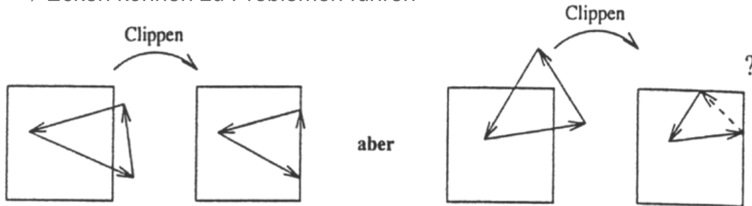
Abb.: Einfügen von Fenstergrenzen beim Polygon-Clipping
