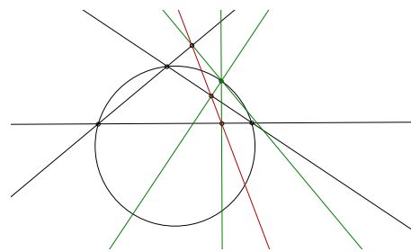
Die Simsonsche Gerade
