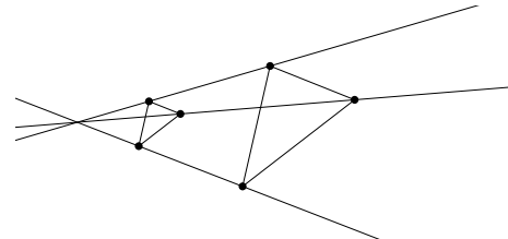
Der (affine) Satz von Desargue
