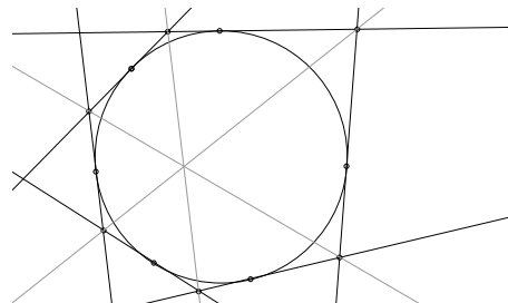
Der Satz von Brianchon
