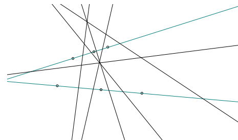
Die 6 Pappusgeraden zu einer Punktkonfiguration
