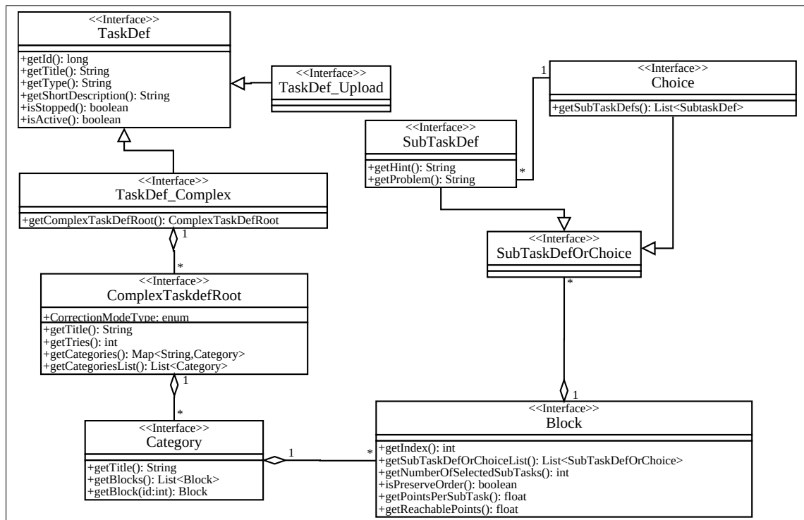
Abbildung 19: ComplexTaskDef-Klassendiagramm
