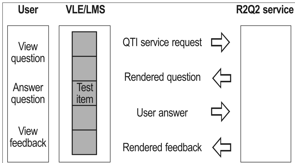
Abbildung 3: R2Q2 Übersicht, Quelle: [wil06b]
