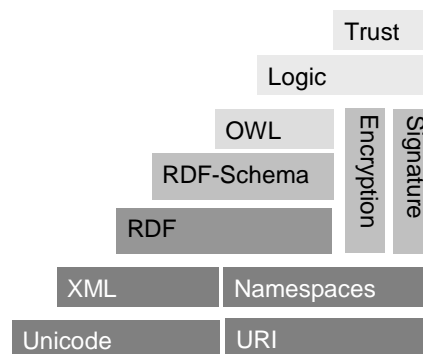
Abbildung 1: Semantic-Web Schichtenmodell [W3C01]
