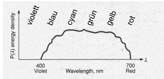
Sichtbarer Frequenzbereich
